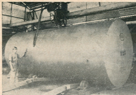
Tanque para almacenamiento de combustible, tipo subterráneo, de 5.200 galones.
